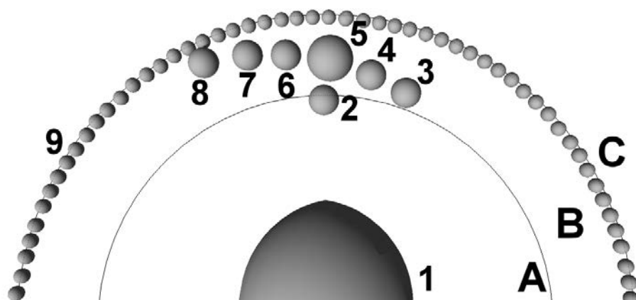
i.61-Cercurile Planetare în Panteon: 1-Oul pământului; A-cercul lunii; B-cercul planetelor; C-cercul stelelor fixe; 2-Luna; 3-Mercur; 4-Venus; 5- Soarele; 6-Marte; 7-Jupiter; 8-Saturn; 9-stelele fixe.
